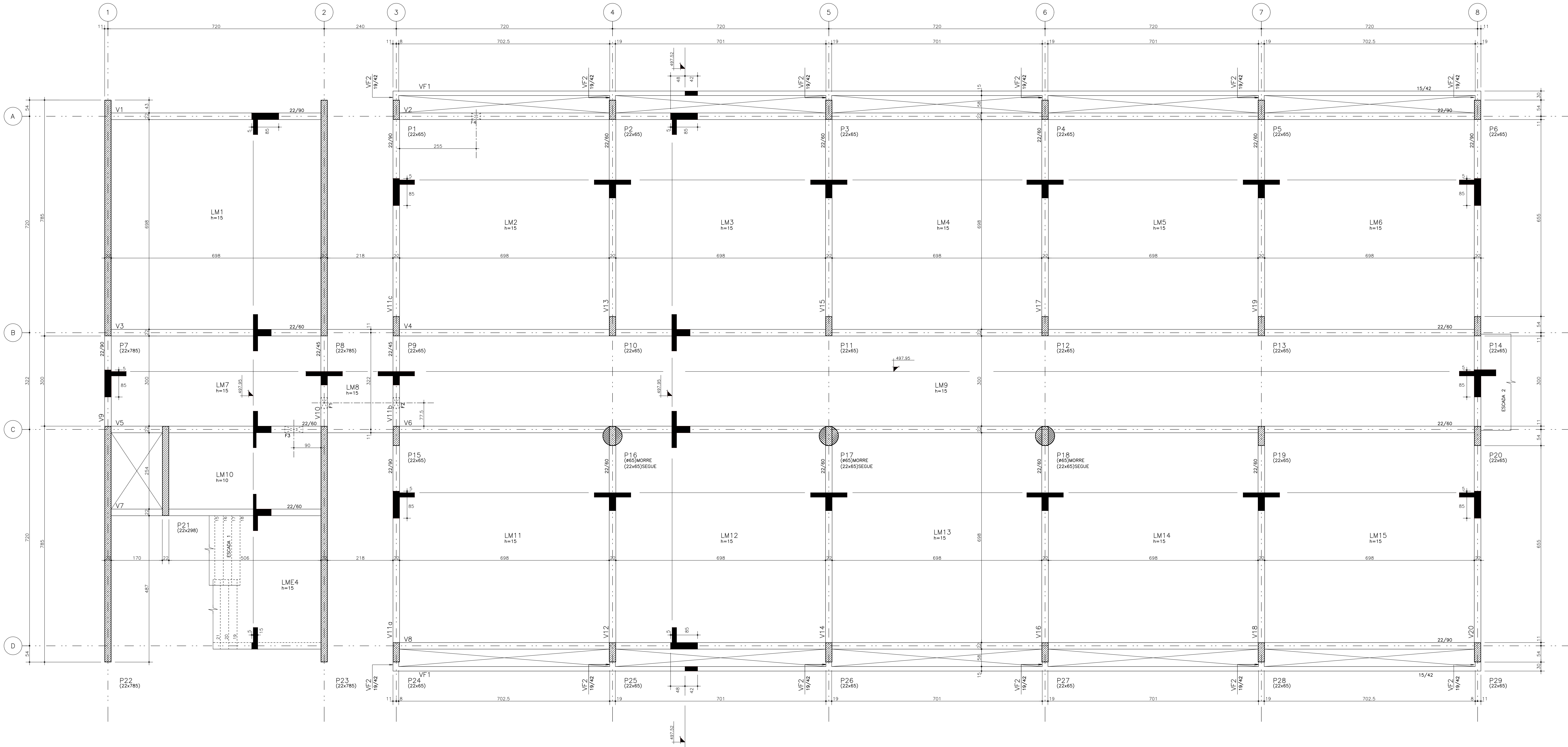
FORMAS DO PRIMEIRO PAVIMENTO ESC. 1:50
